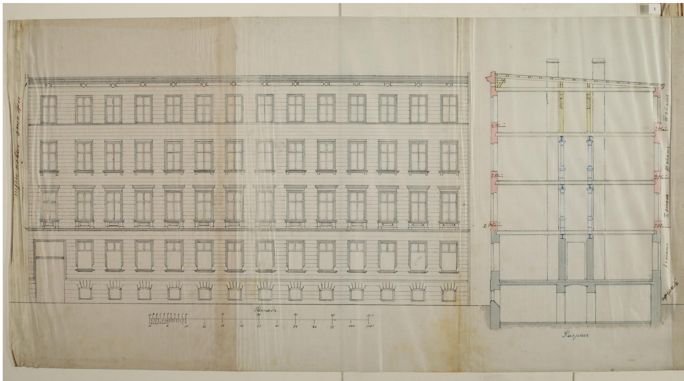
Rūpnīcas galvenā fasāde (pret Aizsargu ielu (tagad Bruņinieku) ielu).
