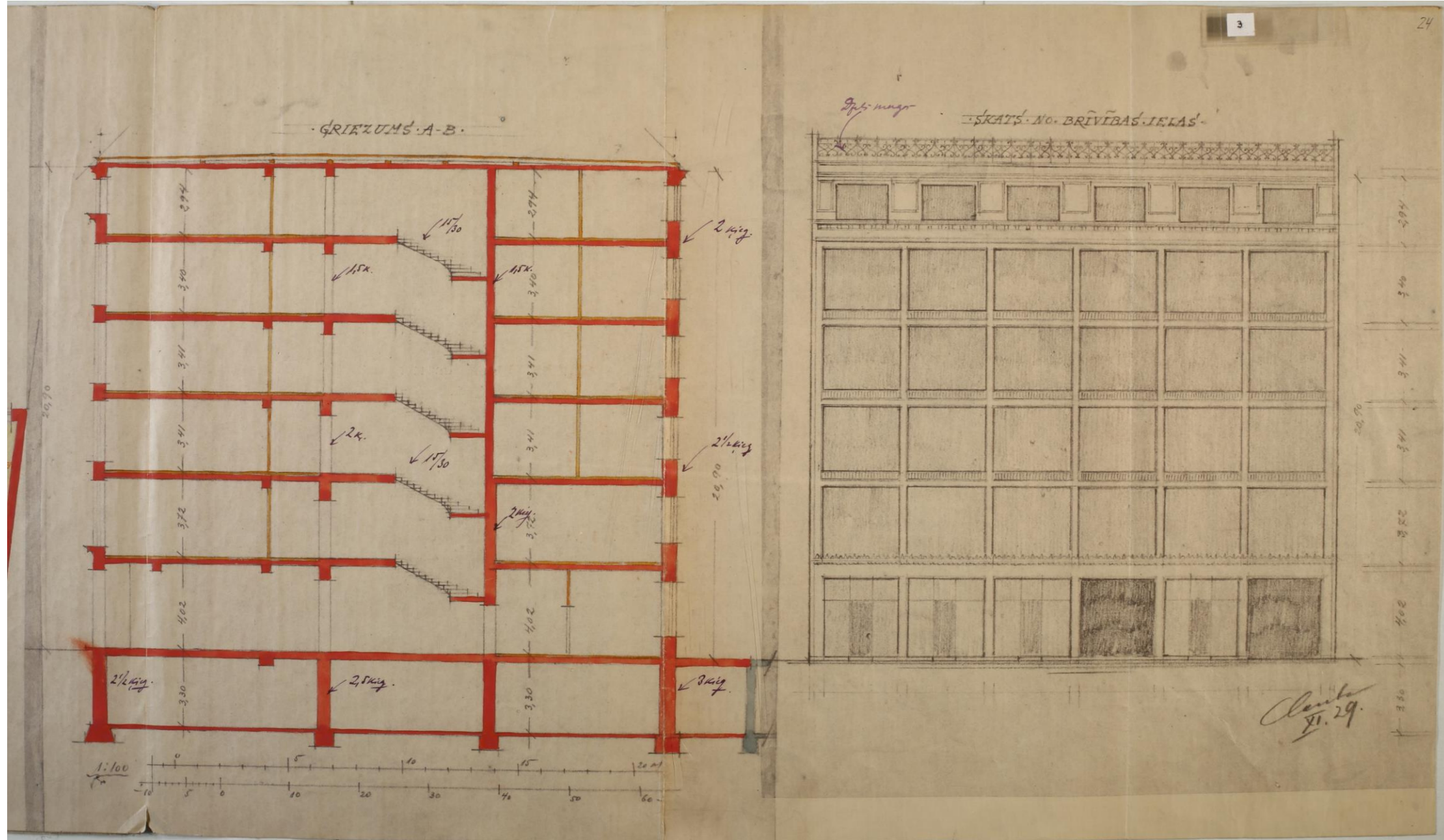
Nama galvenā fasāde un griezums.
