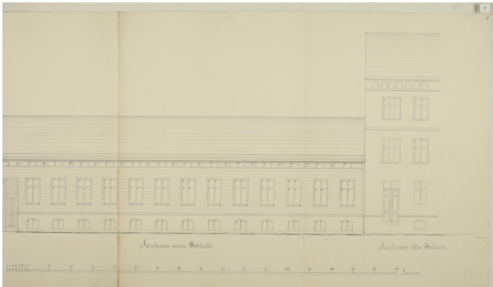
Rūpnīcas noliktavas galvenā fasāde (pret Aizsargu ielu (tagad Bruņinieku) ielu).
