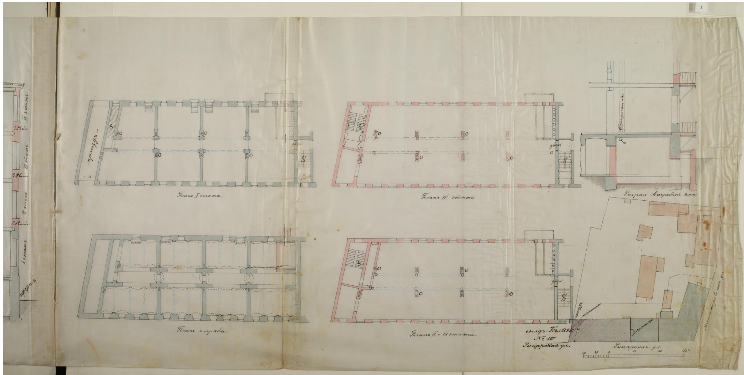
Rūpnīcas piebūves būvprojekta plāni.
